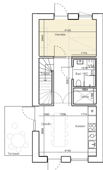
Stueplan Tilvalg 1
