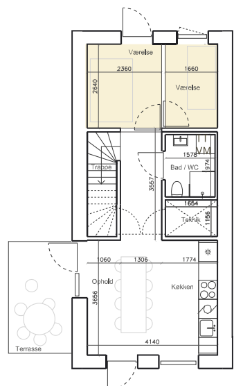
Stueplan Tilvalg 3
