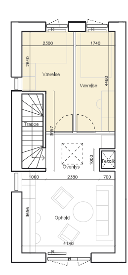
1. sal Tilvalg 1
