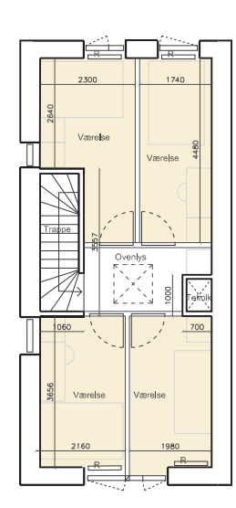
1. sal Tilvalg 2
