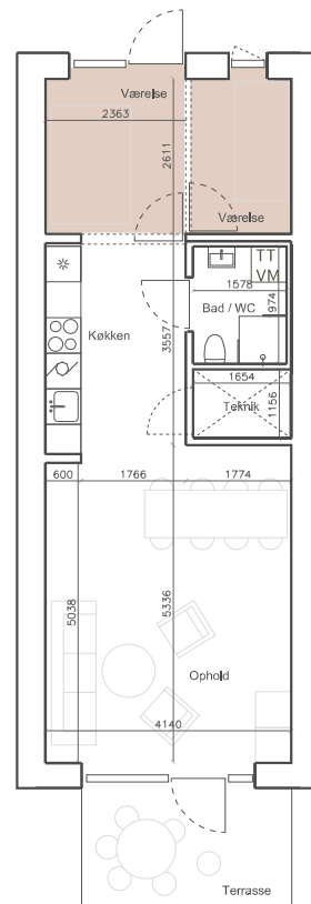
Stueplan Tilvalg 1
