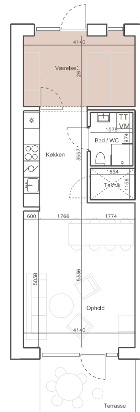
Stueplan Tilvalg 2
