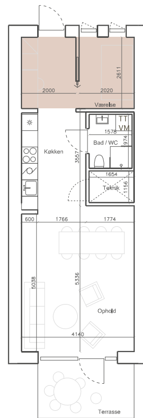
Stueplan Tilvalg
