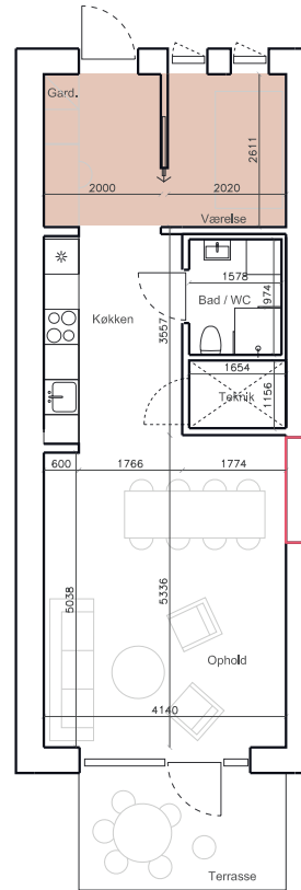
Stueplan Tilvalg
