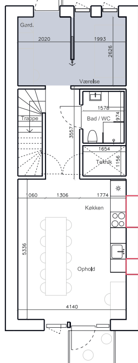
Stueplan Tilvalg 1
