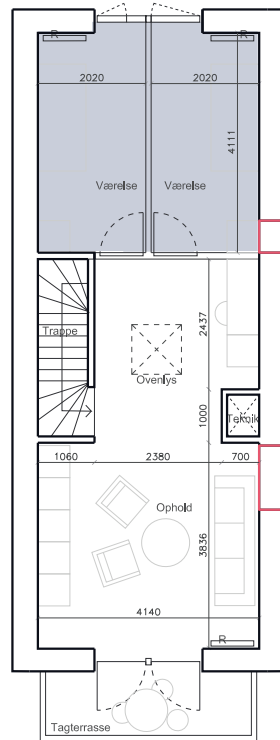
1. sal Tilvalg 1
