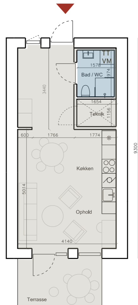
Stueplan, nr. 2 Type A
